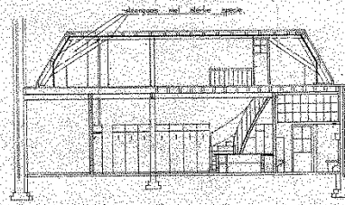
DOORSNEDE A.B.
